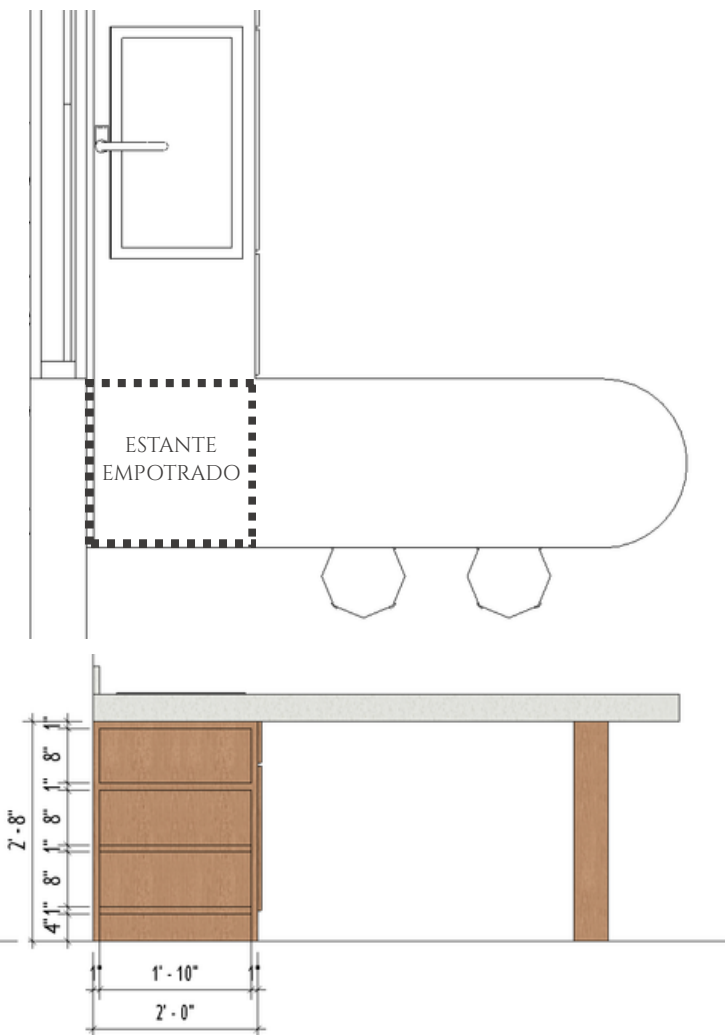
VISTA DE PLANTA (SUPERIOR)
