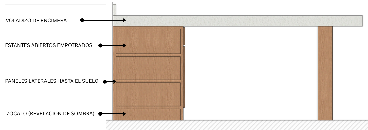
ELEVACION - VISTA FRONTAL
